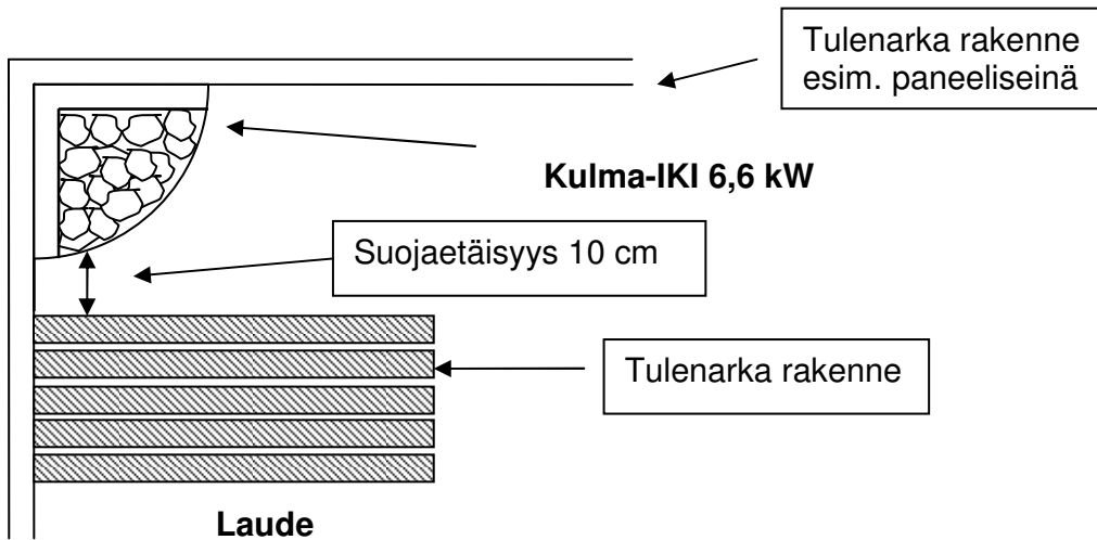
Kuva 1) Kiukaan sijoittaminen nurkkaan ja suojaetäisyydet
